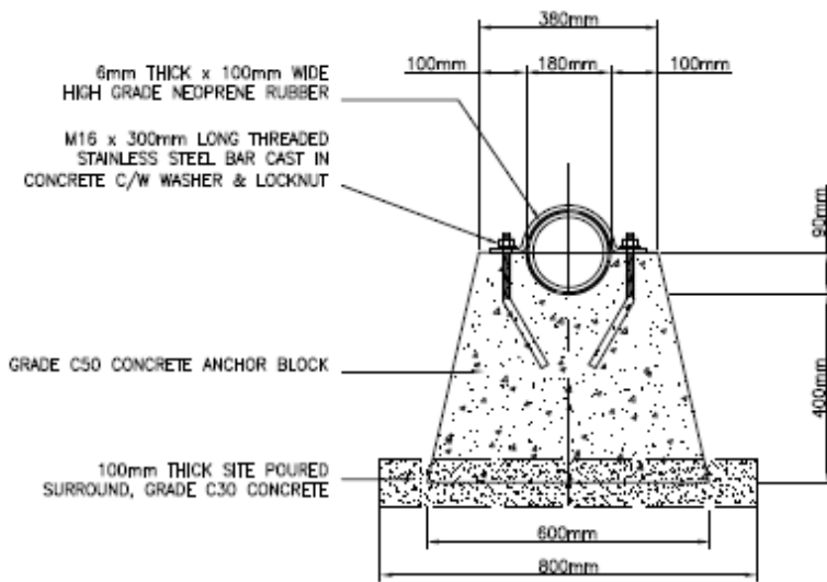
END ELEVATION
