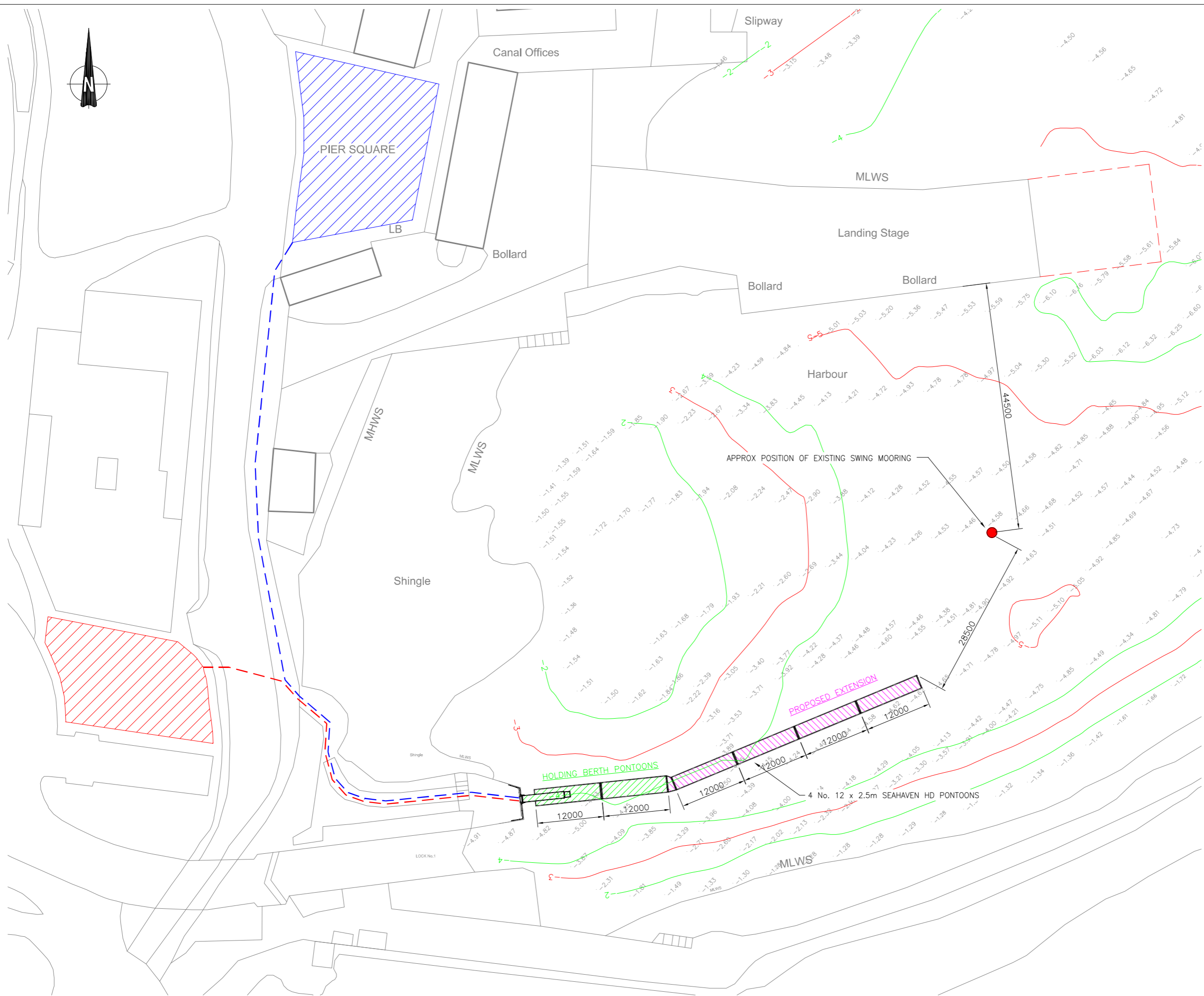
PONTOON LAYOUT
